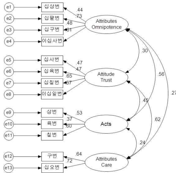
[그림2] 확인적 요인분석 모델
